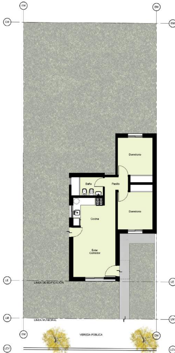
TIPOLOGÍA PLAN 1 Esc.: 1: 100
